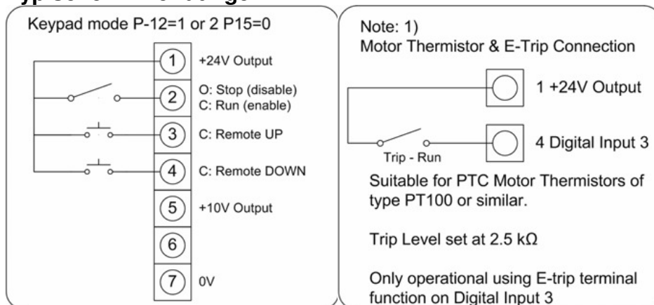
Drehzahl-Tastensteuerung
